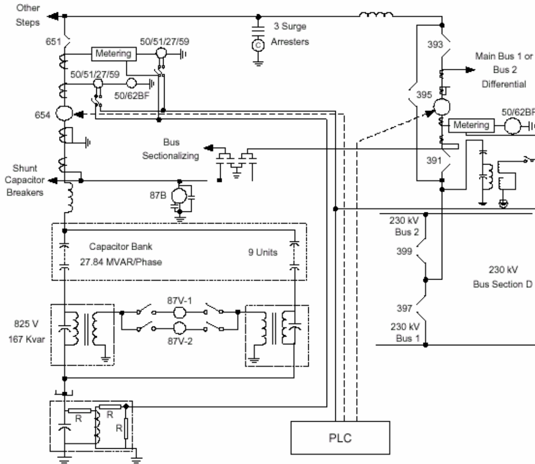
Figura 4: Diagrama Unifilar de um Bloco de Banco de Capacitores sem Fusível com potência nominal de 83.52 MVAR.
