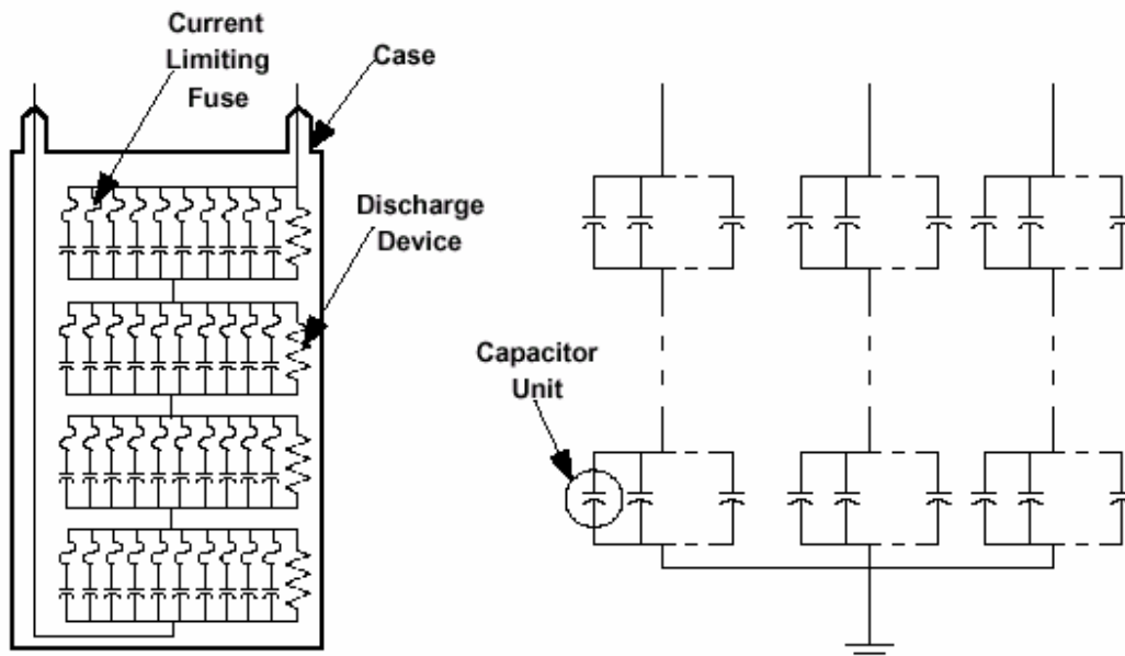
a. Unidade Capacitiva com Fusível Interno
