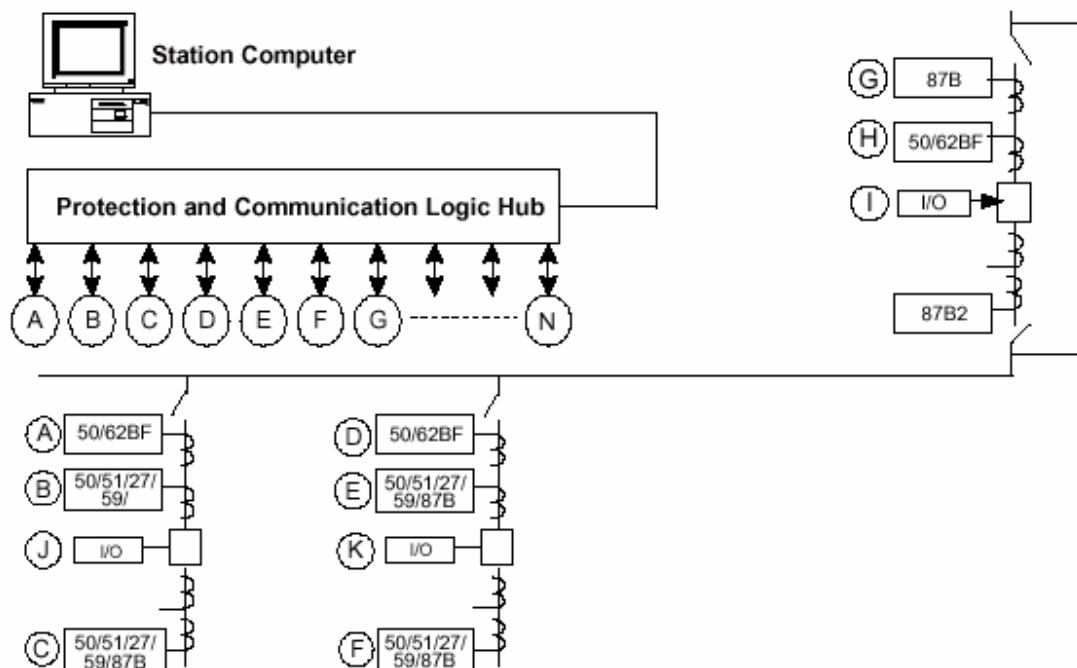
Figura 5: Proteção Futura de Capacitor em derivação, Controle, e Projeto de Esquema Alternativo de Monitoração.
