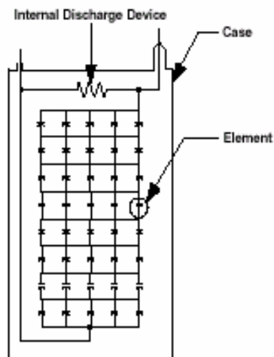
Figura 3a: Unidade Capacitiva sem Fusível
