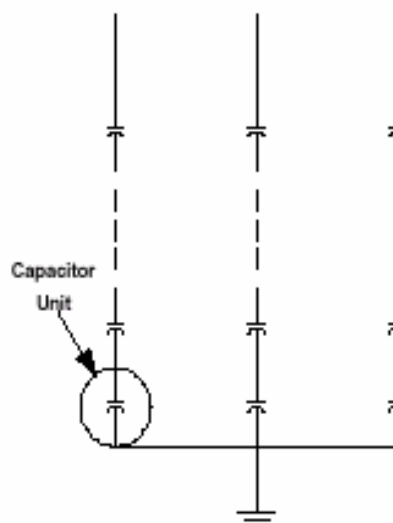
Figura 3b: Banco de Capacitores sem Fusível
