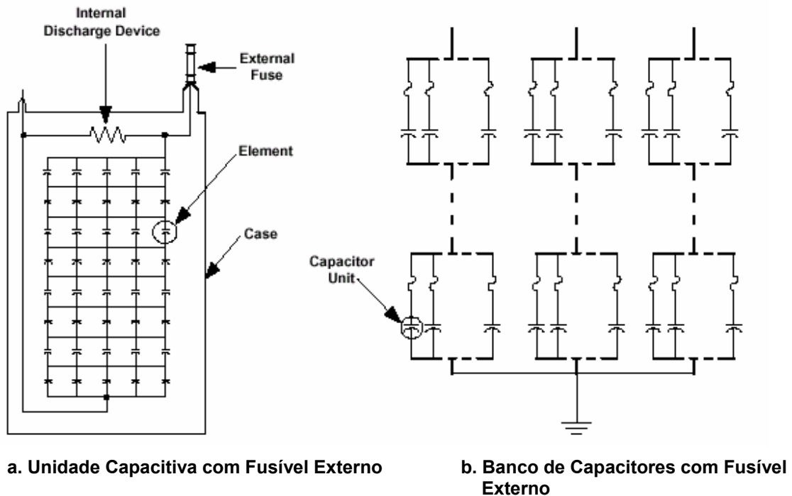
Figura 1: Capacitores de Potência com Fusível Externo
