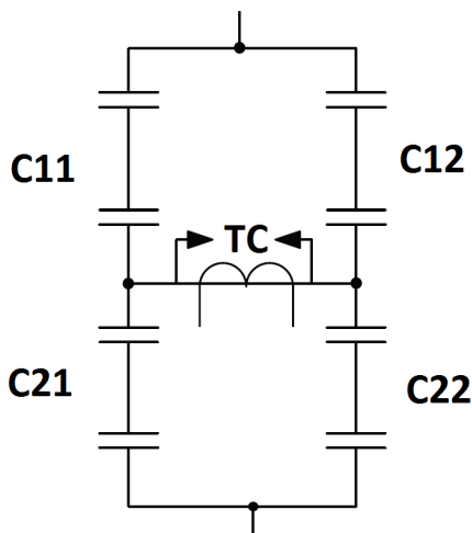
Figura 4 – Arranjo em Ponte-H, somente uma fase mostrada
