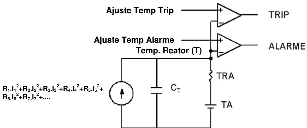
Figura 5 – Modelo Térmico Para proteção dos Reatores de Núcleo de Ar
