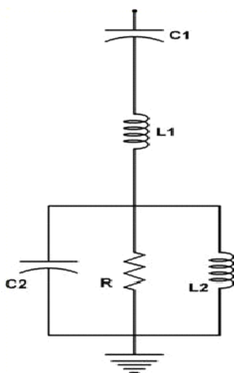
Figura 1 – Arranjo do Filtro de Dupla Sintonia, 3º e 5º Harmônicos
