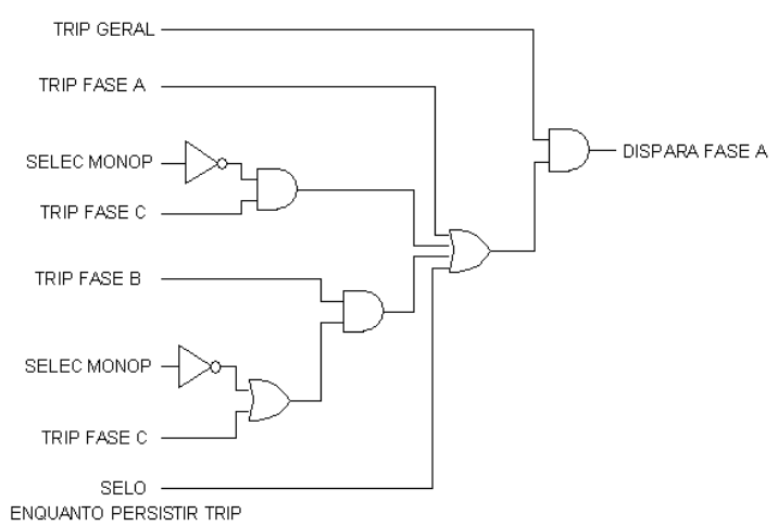
Figura 7 – Lógica Disparo Monopolar Fase A (Similar Para as Fases B e C)
