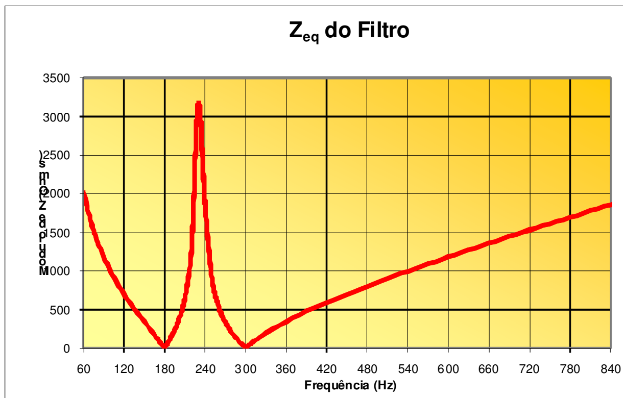
Figura 2 – Impedância Equivalente do Filtro em Função da Frequência
