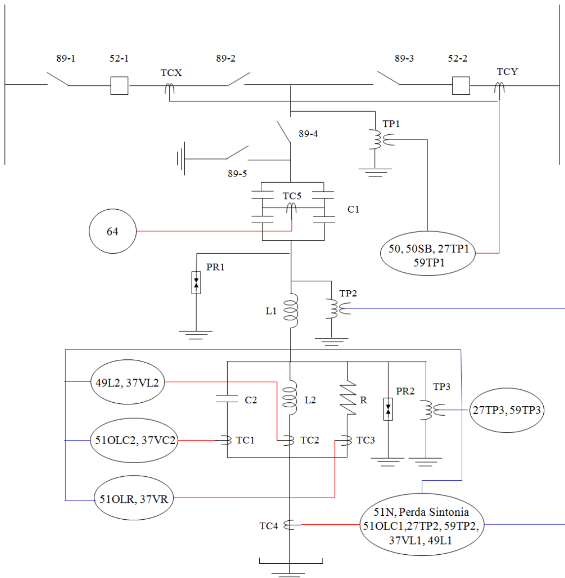
Figura 3 – Conjunto de Funções de Proteção do Filtro
