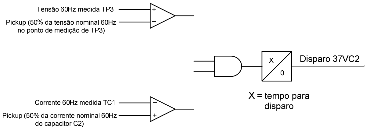
Figura 6 – Lógica da função de subcorrente controlada por tensão
