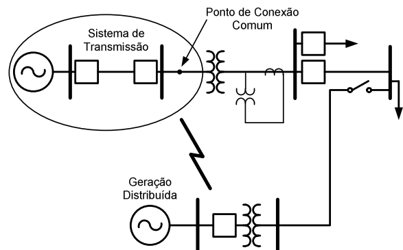
Fig. 2. Proteção da Geração Distribuída
