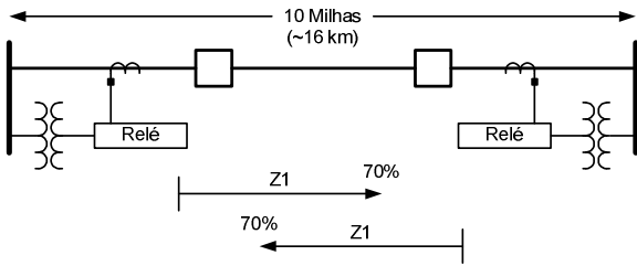
Fig. 3. Proteção Sem Comunicação
