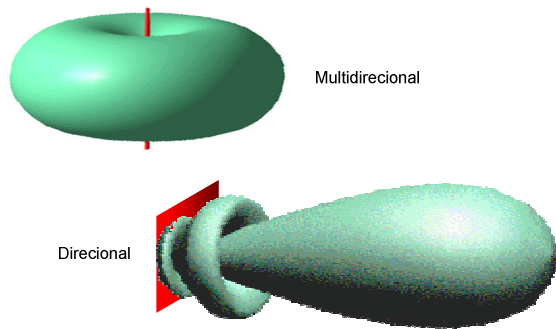
Fig. 10. Antenas Direcionais e Onidirecionais (Multidirecionais)
