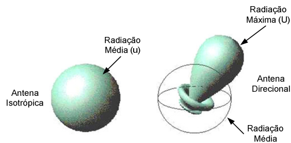
Fig. 11. Ganho da Antena Direcional
