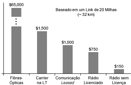
Fig. 23. Comparações de Custos Por Milha para Comunicação
