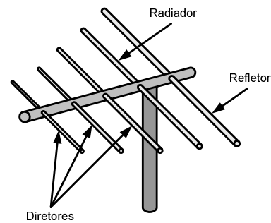
Fig. 12. Antena Yagi
