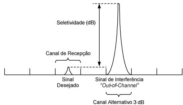
Fig. 9. Seletividade do Receptor
