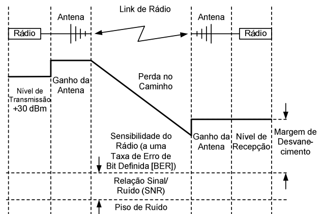
Fig. 7. Link de Rádio Ponto-a-Ponto
