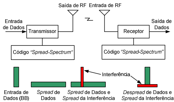
Fig. 18. Ganho no Processamento do Sinal de Interferência do DSSS
