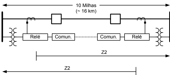
Fig. 4. Proteção Com Comunicação
