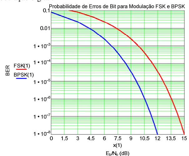
Fig. 8. BER Versus E_b/N_0 para Modulação FSK e BPSK
