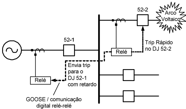
Fig. 6 Use a Comunicação Digital Relé-Relé para Coordenação da Proteção
