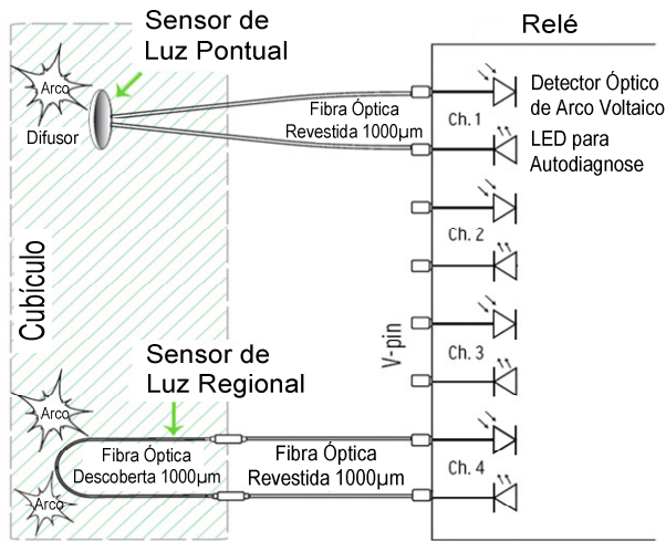
Fig. 7 Esquema de Autodiagnose do Sistema de Detecção de Arco Voltaico com Sensores de Luz Pontuais e Regionais
