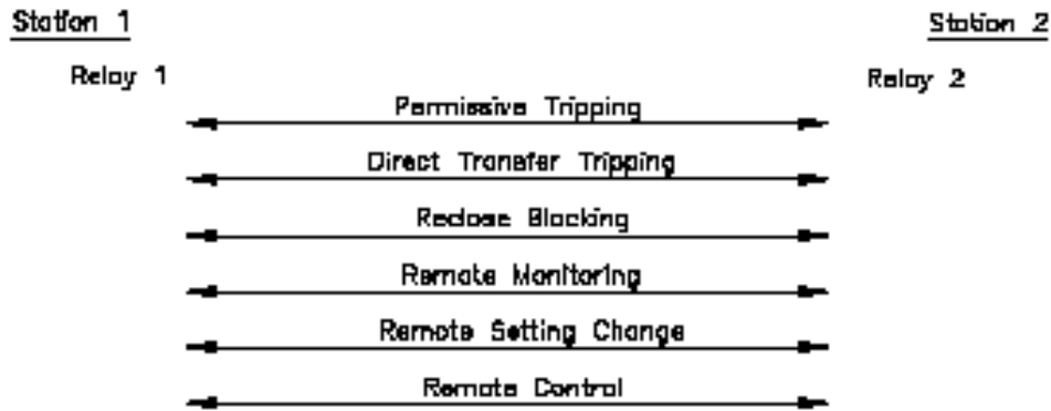
Figura 14: Resumo do Exemplo de Comunicação Lógica Relé-a-Relé
