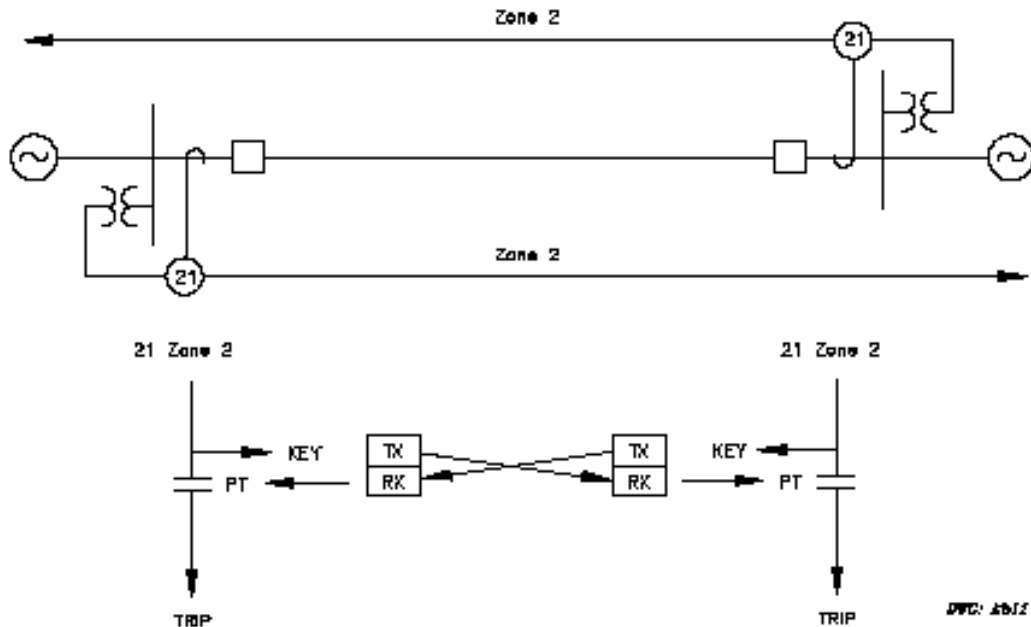
Figura 13: Esquema Básico de Teleproteção com Transferência de Disparo por Sobrealcance Permissivo
