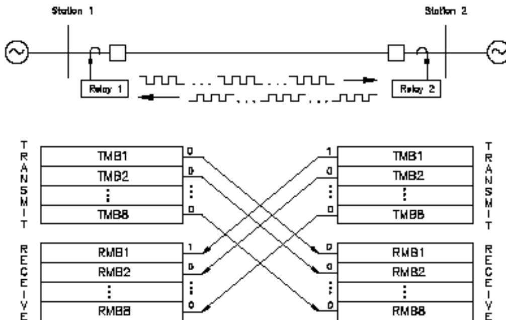
Figura 6: Comunicação Lógica Relé-a-Relé
