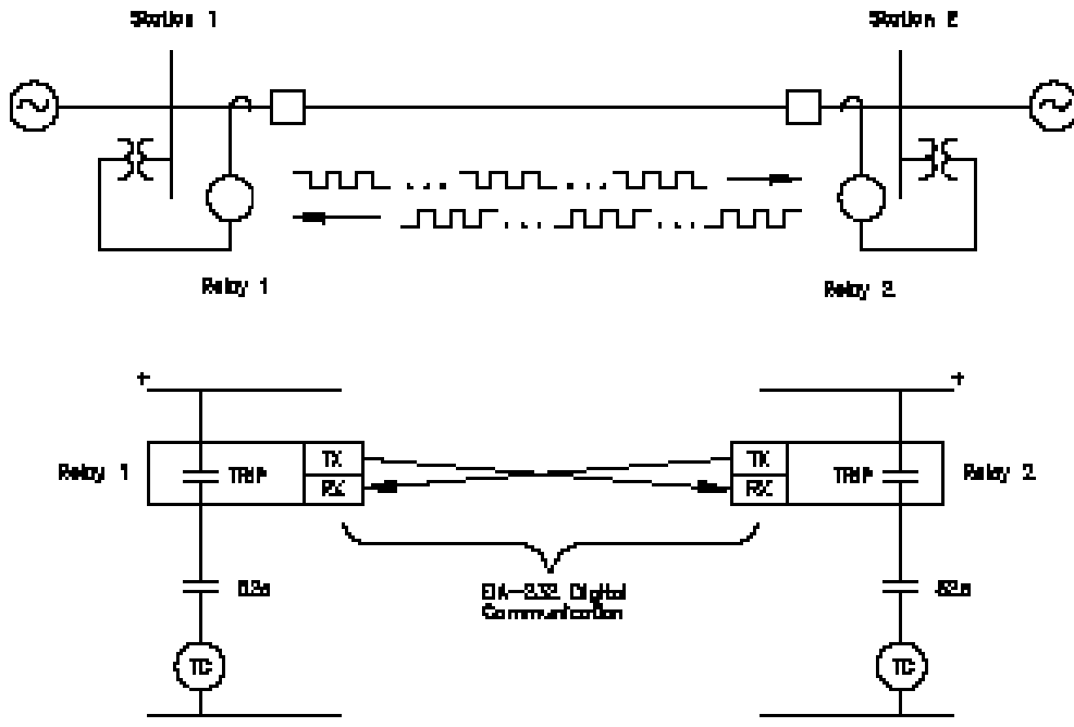
Figura 5: Uma Nova Abordagem : Comunicação Lógica Digital Direta Relé-a-Relé
