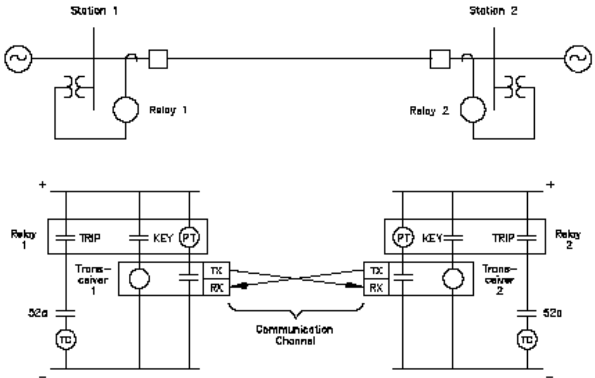
Figure 4: Esquema de Teleproteção de Disparo Permissivo Tradicional com Equipamentos Relé e Comunicação Separados
