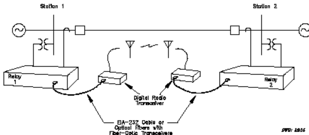
Figura 17: Comunicação Digital via Rádio Digital Ponto-a-Ponto
