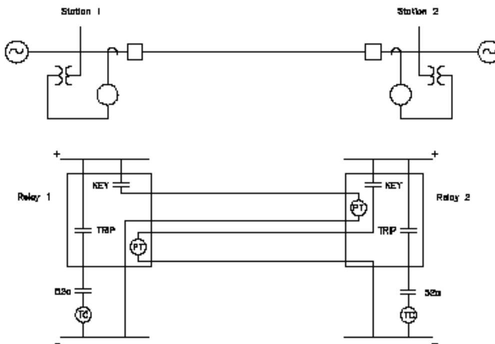
Figura 3: Esquema de Teleproteção de Disparo Permissivo Ideal com Conexões Interligadas
