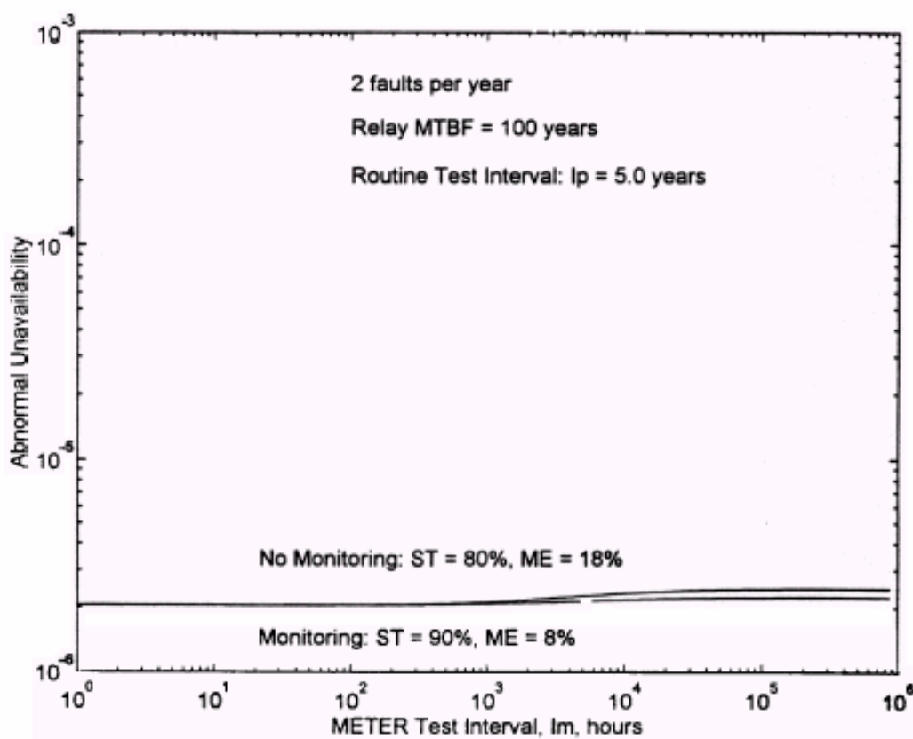
Figura 7 : Uso do monitoramento do sinal AC como um autoteste
