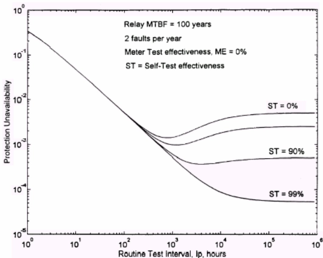
Figura 4: Valores de relés com autoteste
