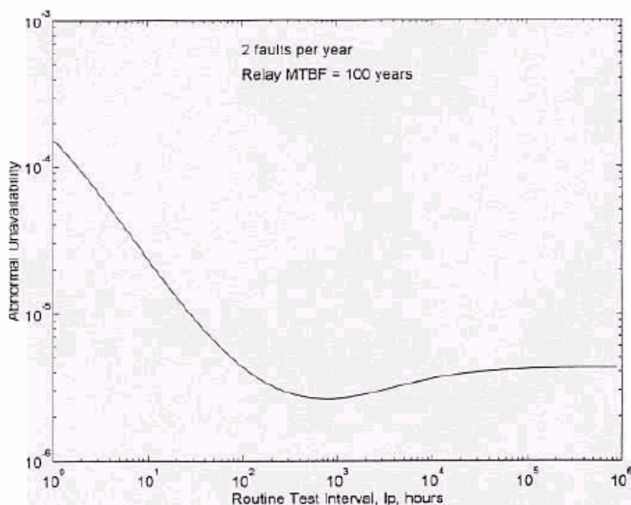
Figura 3 : Intervalo de teste ótimo para relés sem autoteste
