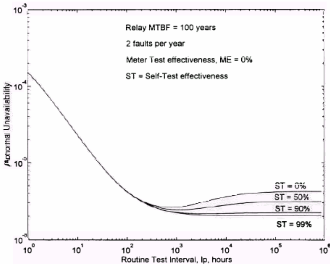
Figura 5: Valores de relés com autoteste
