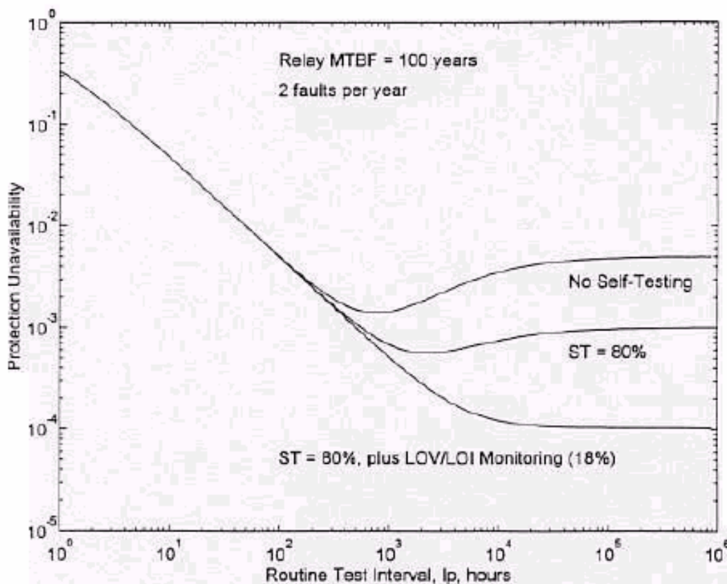
Figura 8: Comparação dos benefícios da adição de autotestes e perda do sinal de monitoramento.
