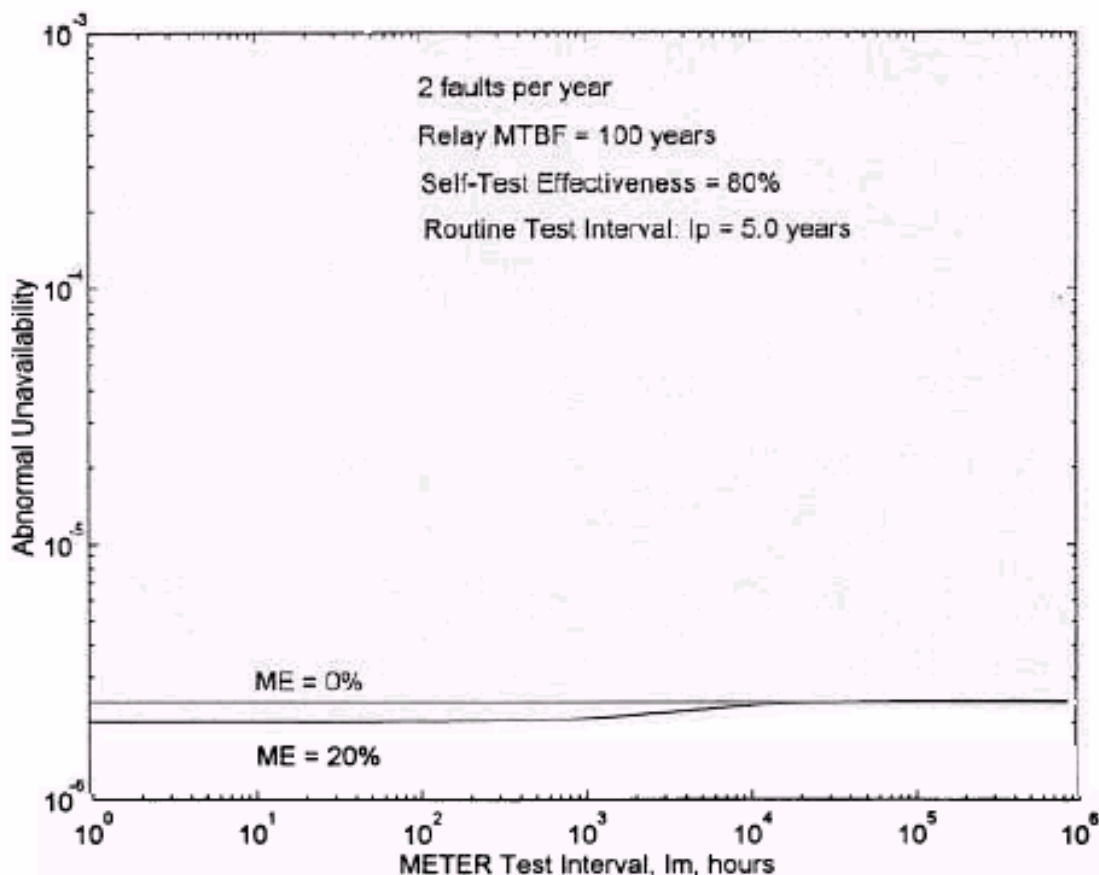
Figura 6 : Benefícios da execução dos testes de medição
